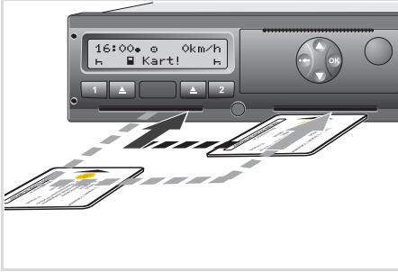
Sürücü kartlarının değiştirilmesi
