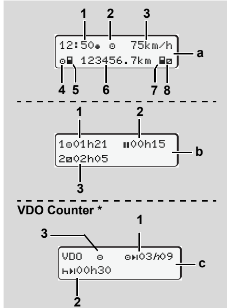
Seyir halindeyken standart göstergeler
