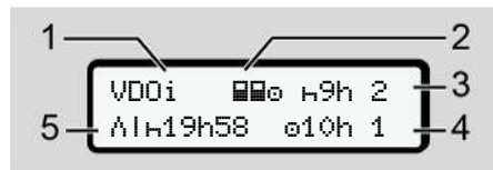
Abb. 73: VDO Counter – Statusanzeige
