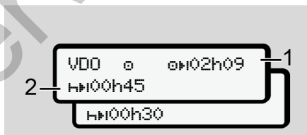
Abb. 60: Aktivität \text{H} – verbleibende Lenkzeit vs. tägliche Ruhezeit
