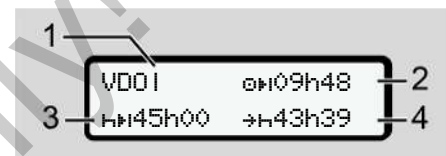
Abb. 71: Aktivität \square / \square – Wochenwerte
