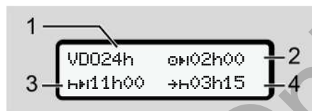
Abb. 70: Aktivität \square / \square – Tageswerte
