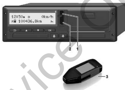
Abb. 12: Anschluss an die Frontschnittstelle
