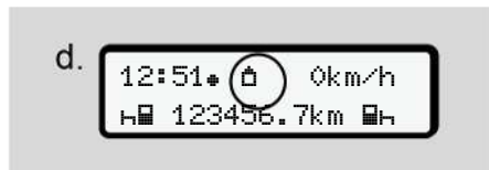
Abb. 46: Standardanzeige mit gesteckter Unternehmenskarte
