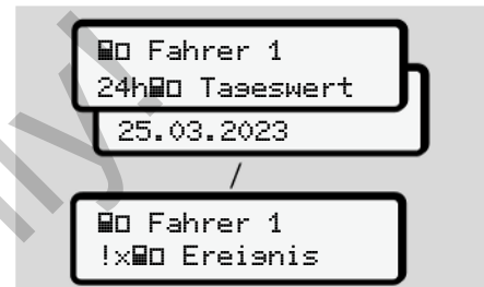
Abb. 125: Menüfolge Anzeige für Fahrer-1
