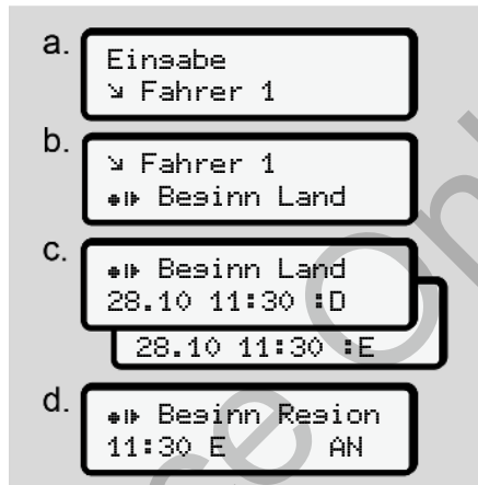
Abb. 96: Menüfolge Eingabe – Beginn Land
