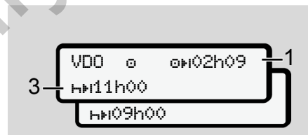
Abb. 61: Aktivität \text{H} – verbleibende Lenkzeit vs. tägliche Ruhezeit
